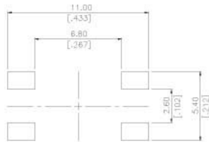
(SCALE 8:1) P.C.B. LAYOUT
