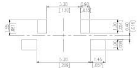
P.C.B. LAOUT
