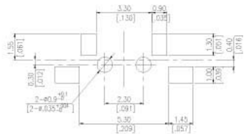
P.C.B. LAOUT
