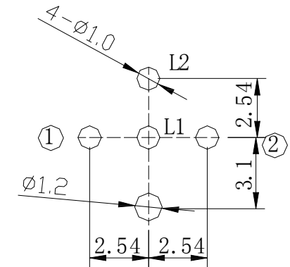
P. C. B. LAYOUT
