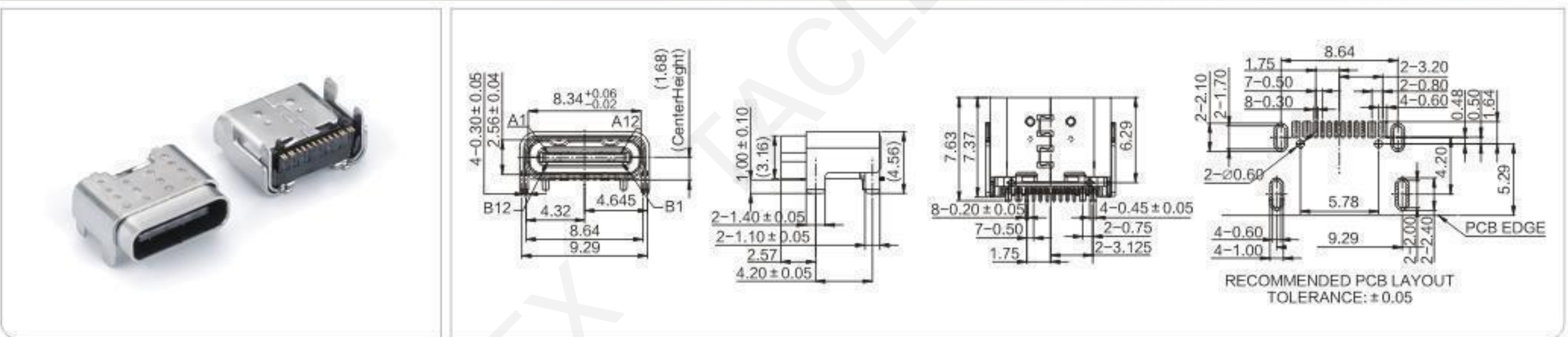
防水TYPE-C F 16P板上四脚插板SMT 7.37L
