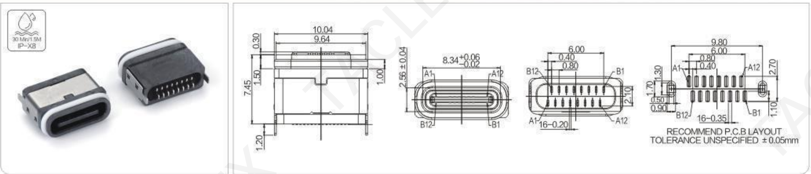
TYPE-C 16P母座防水IPX8 两脚立贴 L=7.6 全塑
