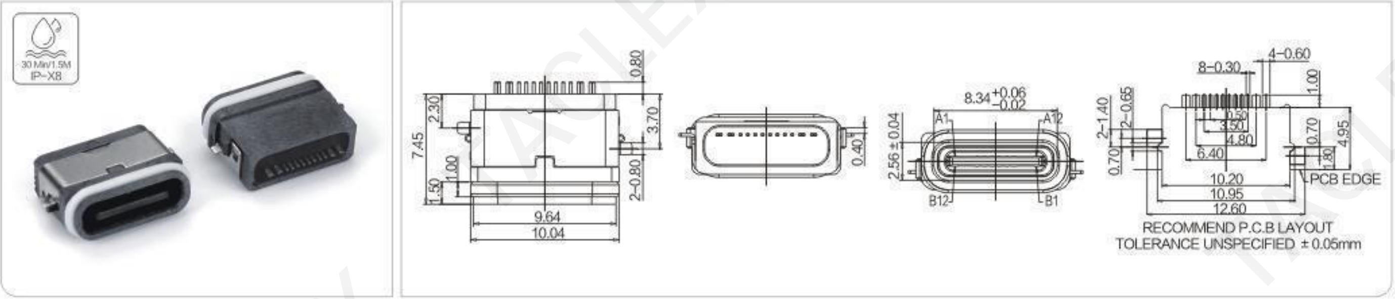
TYPE-C 16母座防水IPX8 沉板 0.8/1.2/1.6 两脚SMT L=7.6 全塑
