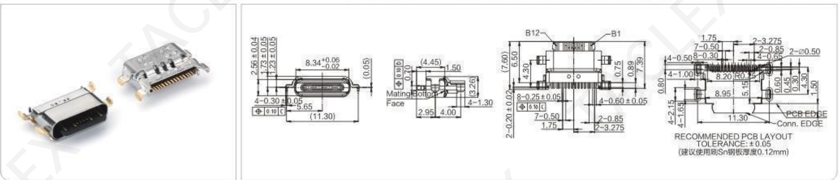
防水TYPE-C F 16P沉板1.53四脚插板SMT 6.1L
