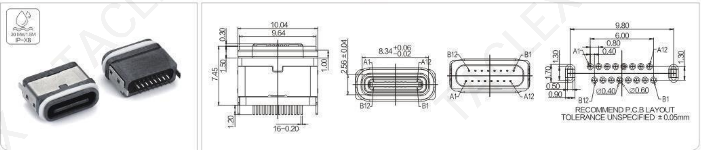
TYPE-C 16P母座防水IPX8 两脚立插 L=7.6 全塑
