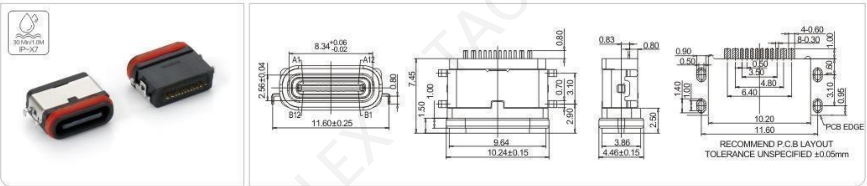
TYPE-C -16P 防水母座沉板0.8 1.2 1.6 L=7
