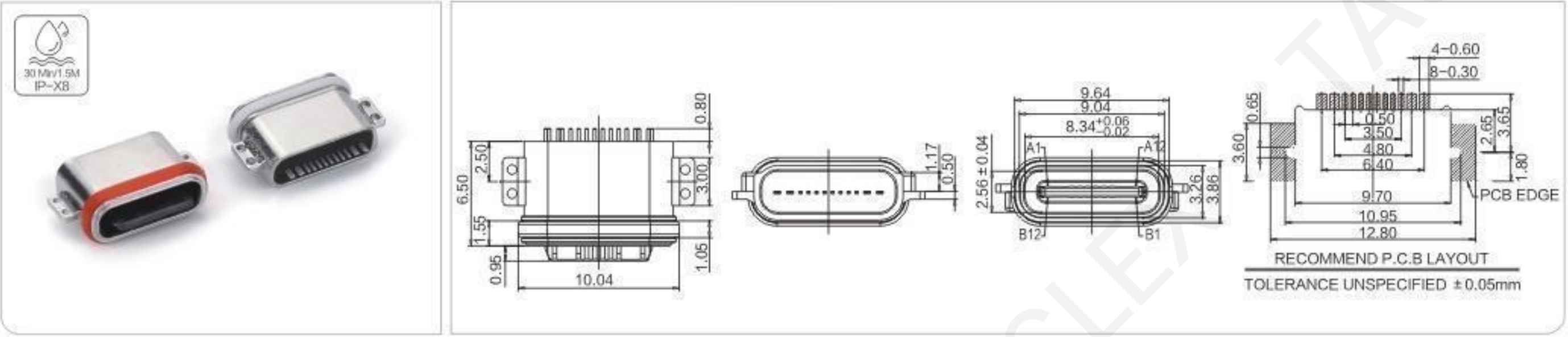
TYPE-C 16P母座防水IPX8 沉板0.8/1.2/1.6 粉末冶金外壳L=6.50 舌头外露0.95
