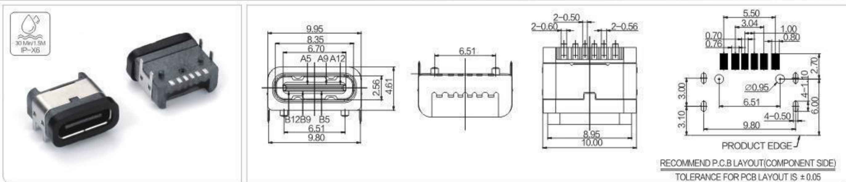
TYPE-C 6P板上防水母座 外壳四脚插板 端子SMT
