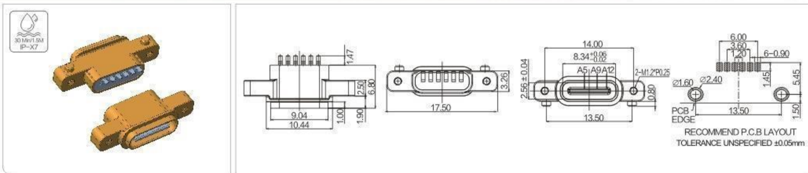
TYPE C 6P 防水母座板上 L=6.8mm (带M1.2螺丝外壳)
