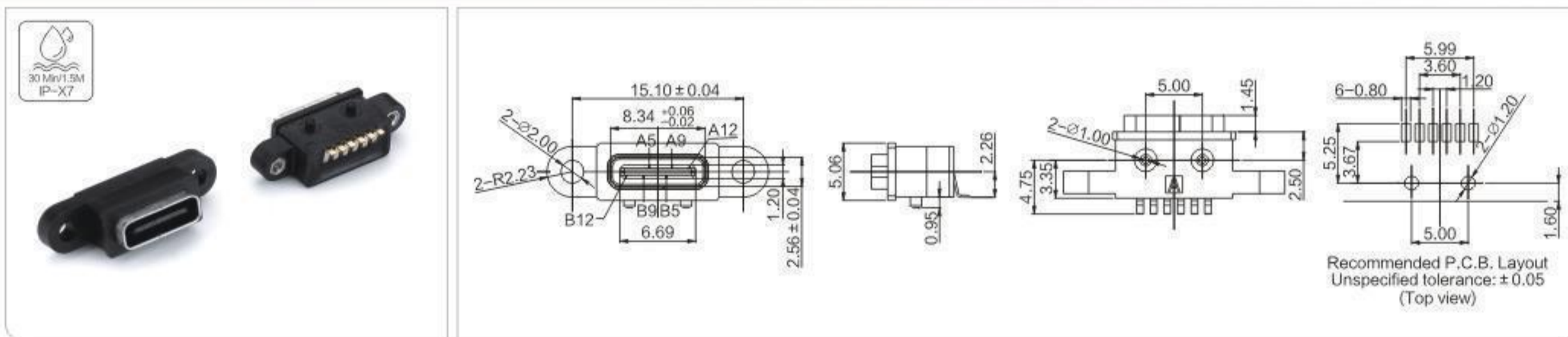
防水TYPE-C F 6P锁壳式SMT 带定位柱 7.3L
