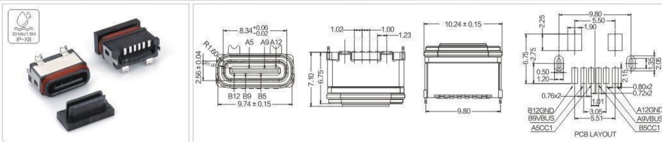
TYPE-C 6PIN母座 直立式贴片 6.8H 全塑防水母座
