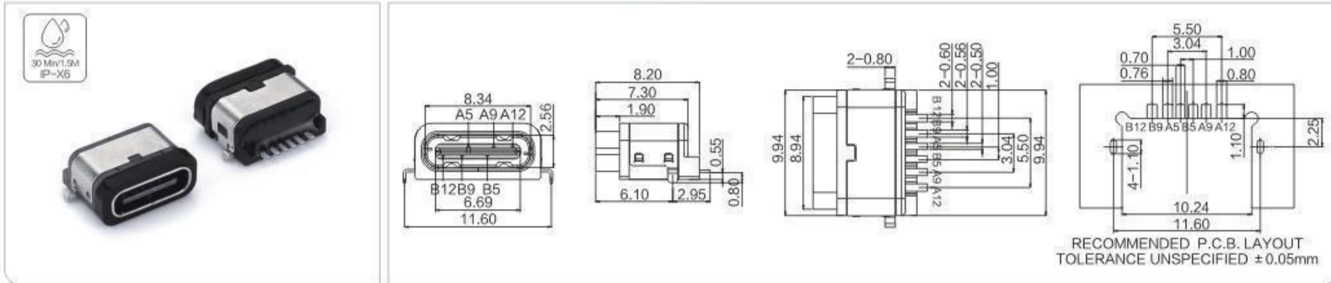
防水TYPE-C F 6P沉板0.55四脚插板SMT 8.2L
