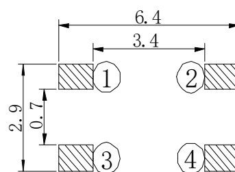
焊接尺寸图
