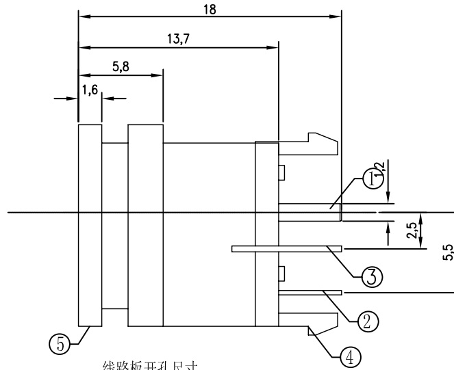
线路板开孔尺寸 P.C.B LAYOUT
