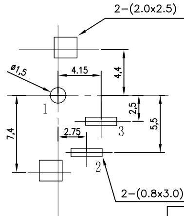
线路板开孔尺寸 P.C.B LAYOUT
